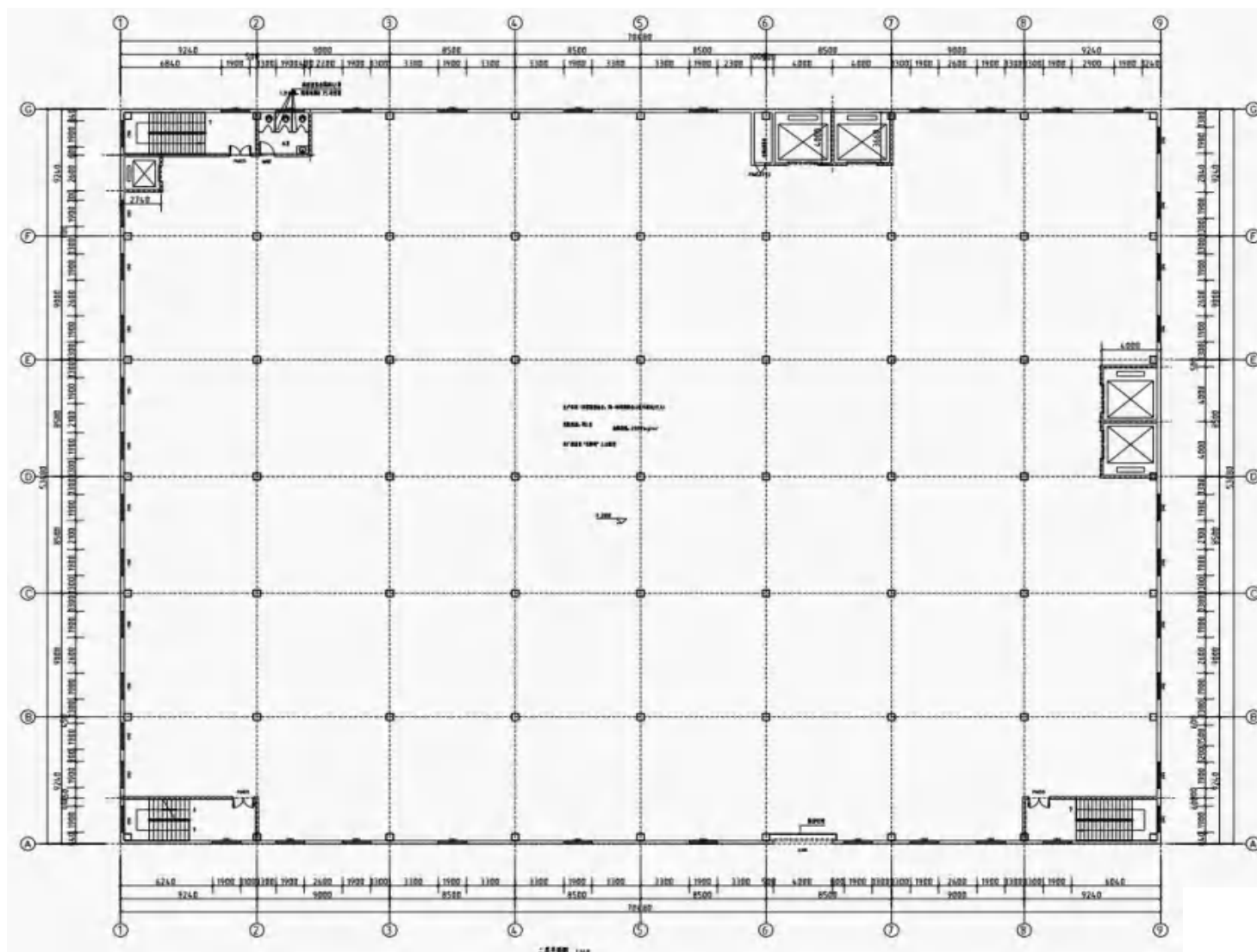
附图 8 厂区平面布置图 (2 层)
