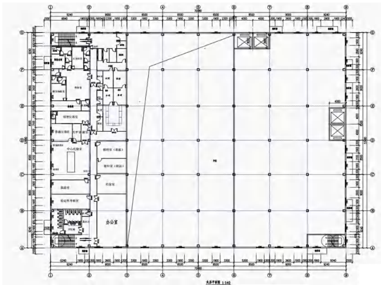
附图 7 厂区平面布置图（夹层）
