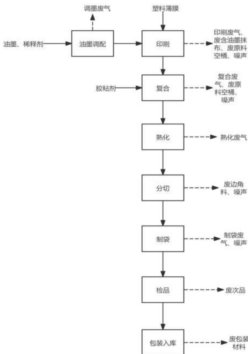
图 2-2 药用复合膜、食品包装膜（袋）生产工艺与产污环节图
